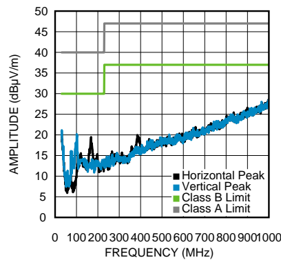
Radiated EMI (EN 55022) V_{IN} = 12V, V_{OUT} = 5V, I_{OUT} = 8A
