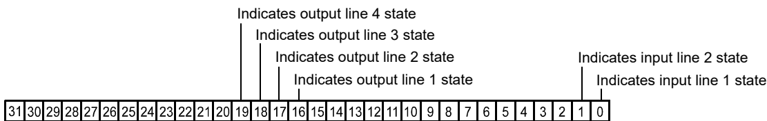
Fig. 73: Line Status All Parameter Bits
