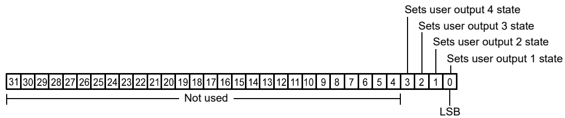
Fig. 27: User Output Value All Parameter Bits
