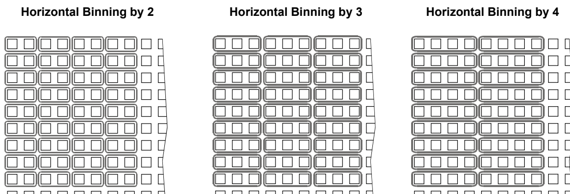
Fig. 64: Horizontal Binning
