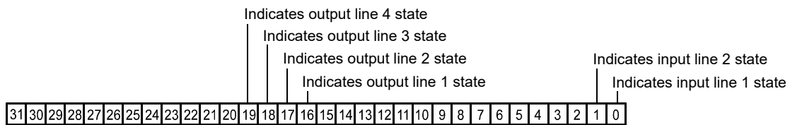
Fig. 29: Line Status All Parameter Bits
