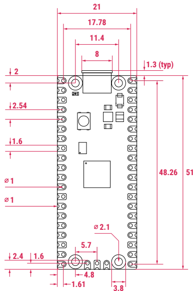
Pico 2
