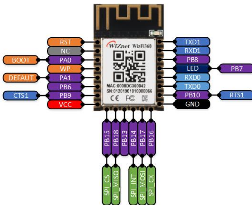
Figure 3. WizFi360 Pinout
