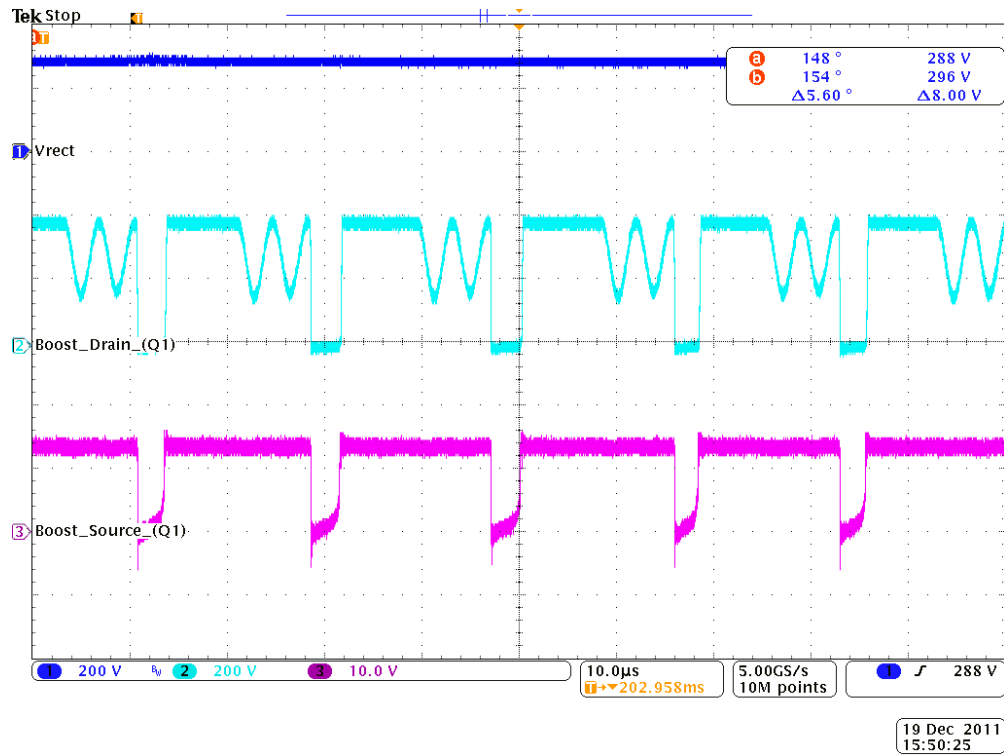
Figure 16. Boost FET, Q1, Waveform
