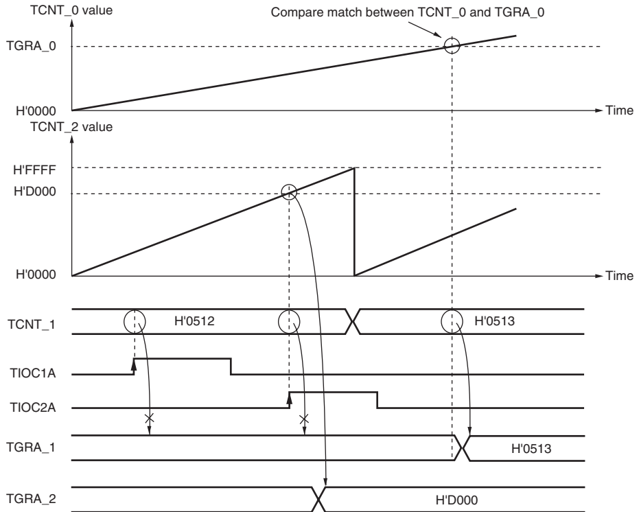
Figure 9.24 Cascaded Operation Example (d)
