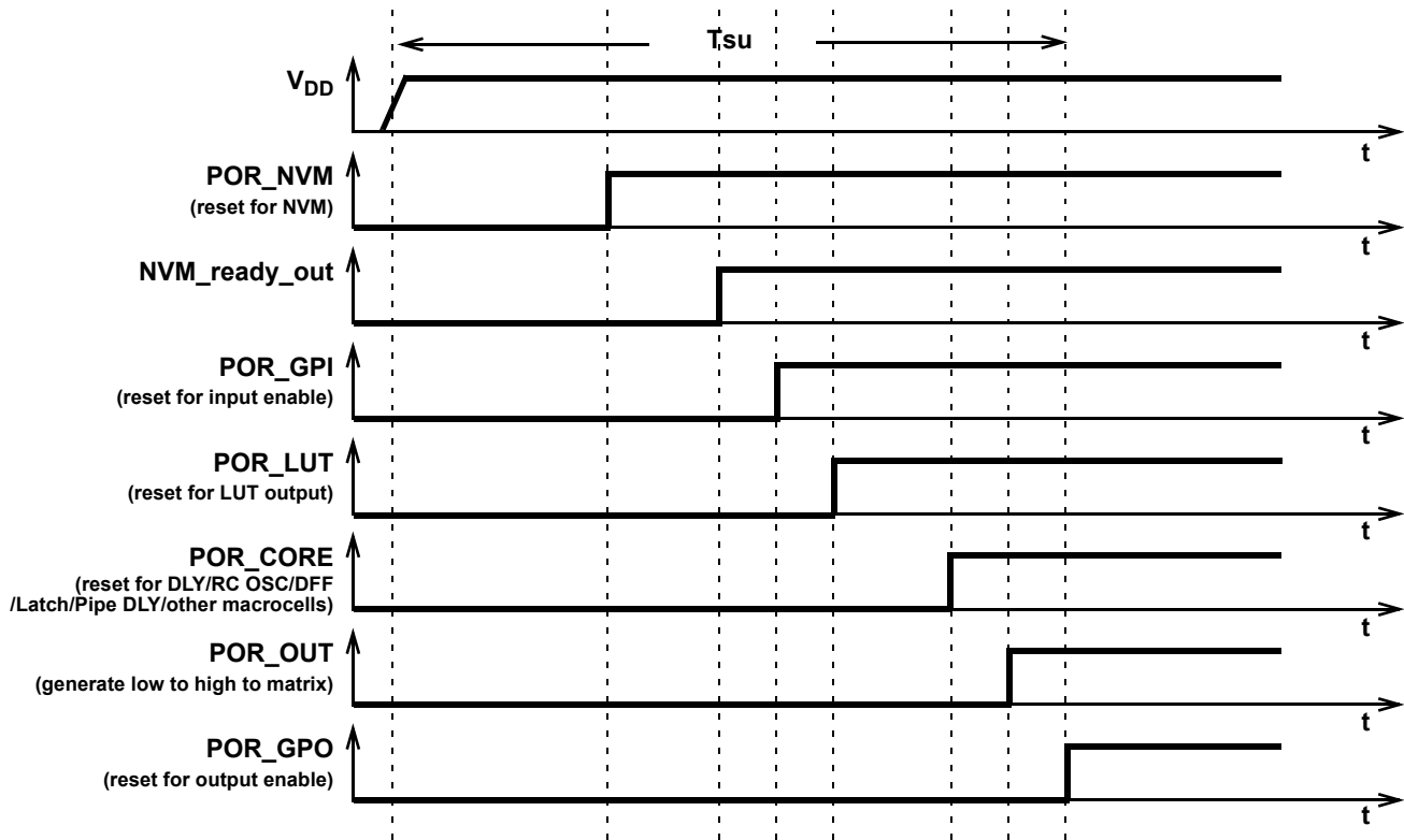
Figure 47. POR sequence
