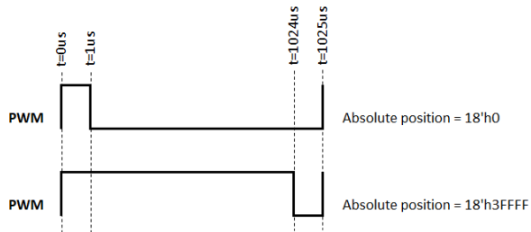
PWM Period: 1025 \mu\text{s}
