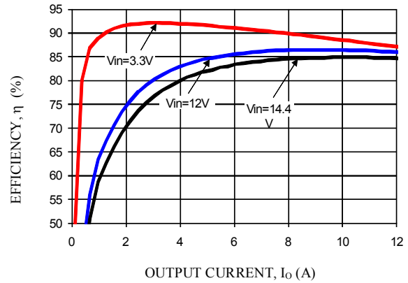
V_o = 1.2V
