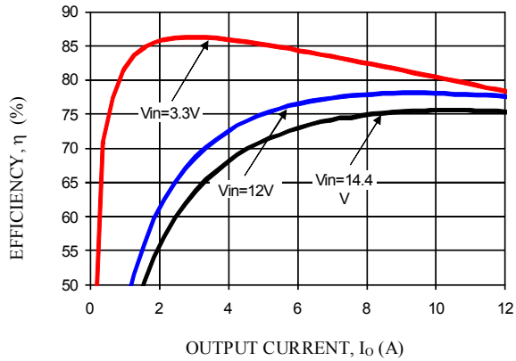
V_o = 0.6V
