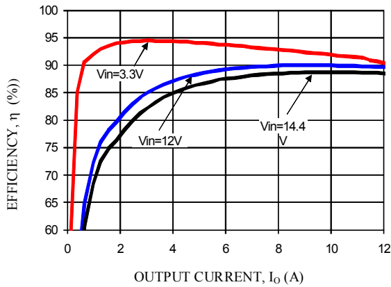
V_o = 1.8V
