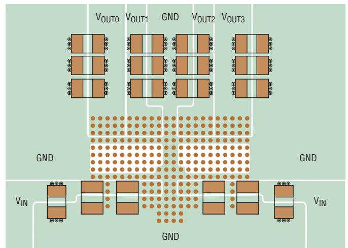
(b) LTM4681 Bottom Layer
