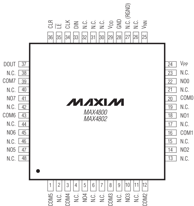
TQFP 7mm x 7mm
