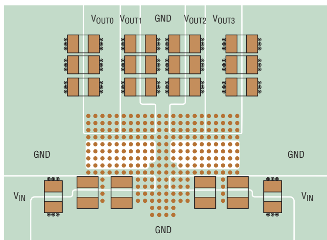
(b) LTM4682 Bottom Layer
