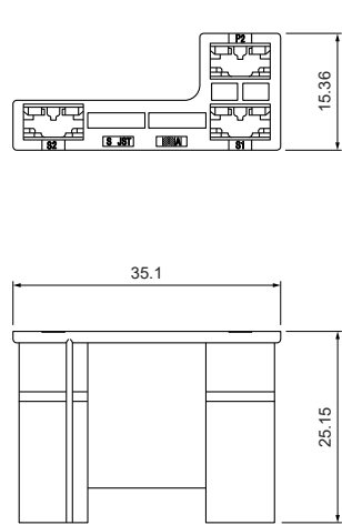
RSFP-3V-ES-B
