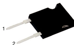
TO-247AC 2L
