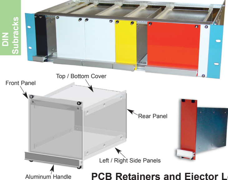
CCA46 to CCA57 for card retainers or DIN Modules
