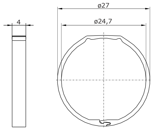
Hauptabmessungen Farbring
