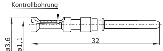
Hauptabmessungen Kontaktstift
