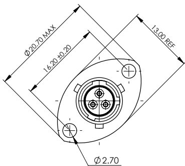
RECEPTACLE - TYPE 0
