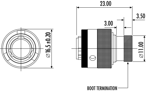
RECEPTACLE - TYPE 0
