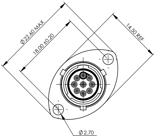
RECEPTACLE - TYPE 0
