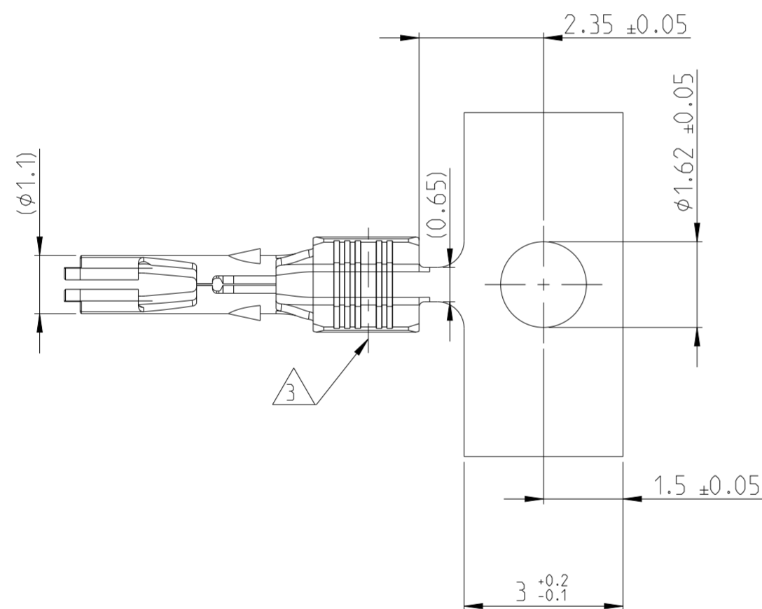
SECTION B-B 20:1
