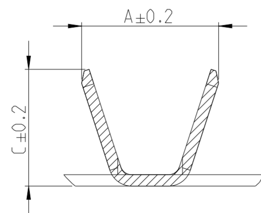
SECTION B-B 20:1
