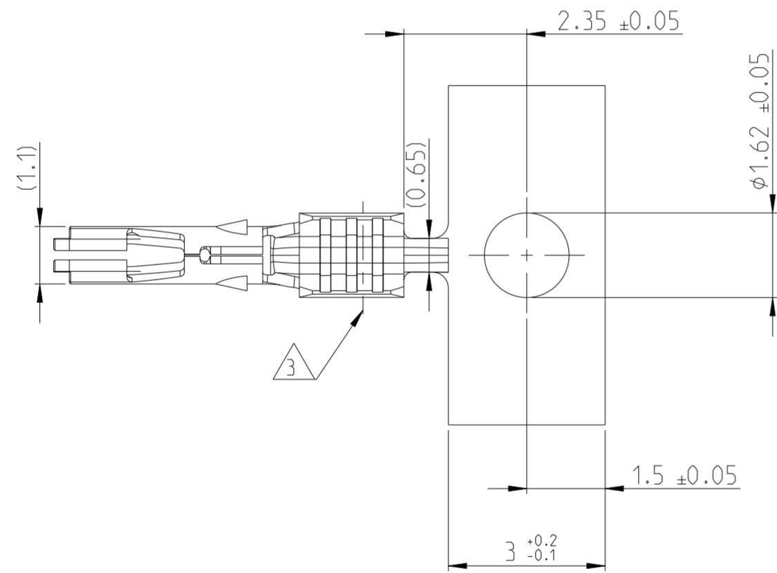
SECTION B-B 20:1
