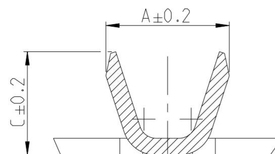
SECTION B-B 20:1
