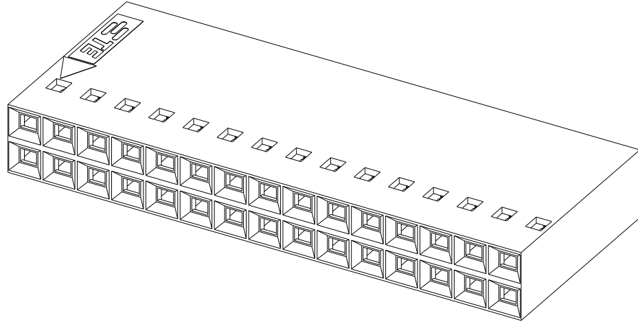
SCALE 3:1
