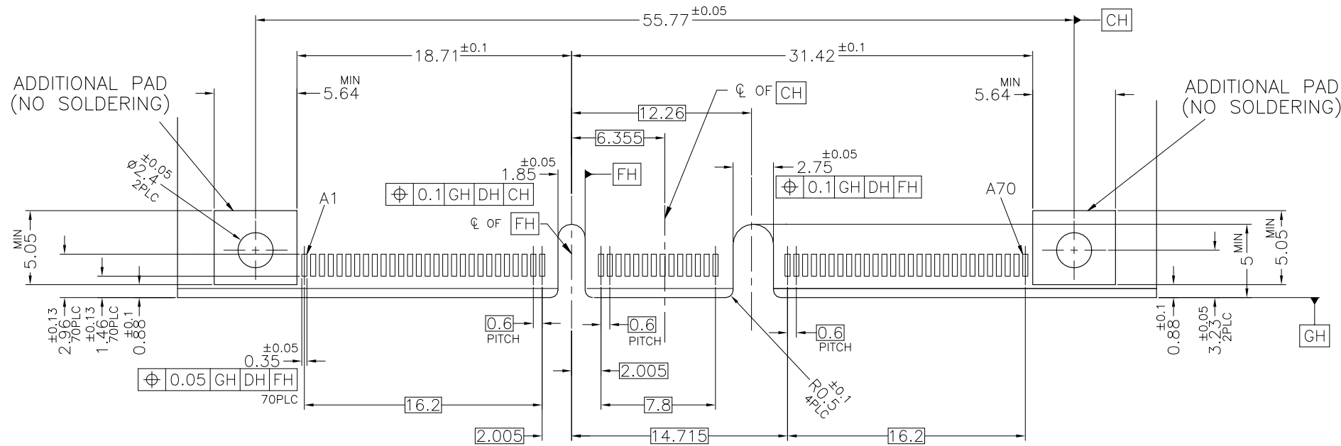
VIEW A-A
