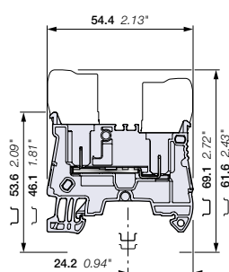
ZD2.5-11
