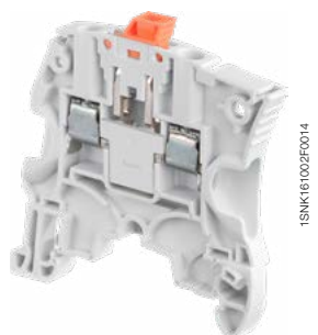
ZS4-S
