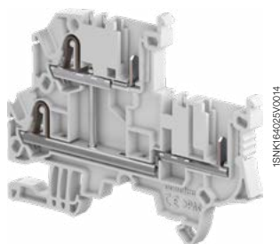
ZDK2.5-D1
