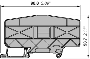
CS-R3
