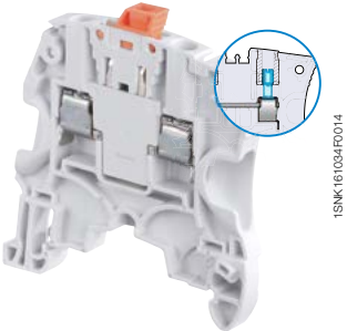
ZS4-S-T
