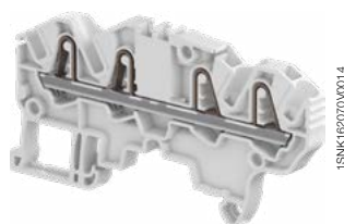
ZK2.5-4P
