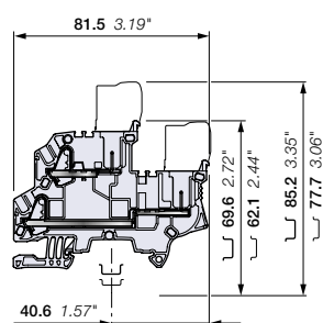
ZDK2.5-D2
