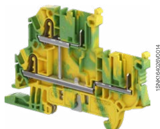
ZDK2.5-D1-PE
