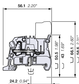
ZDK2.5-11-PE
