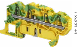
ZK2.5-PE-4P
