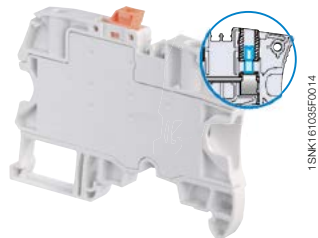
ZS4-S-T-R1
