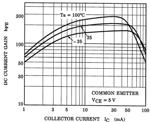
Fig. 10.18 RN1906FE h_{FE}-I_C
