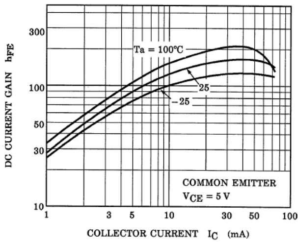
Fig. 10.15 RN1903FE h_{FE}-I_C
