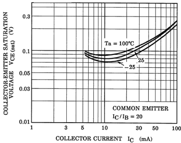
Fig. 10.19 RN1901FE V_{CE(sat)}-I_C
