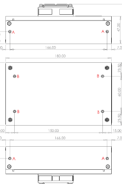
STANDARD CHASSIS + TOP FAN
