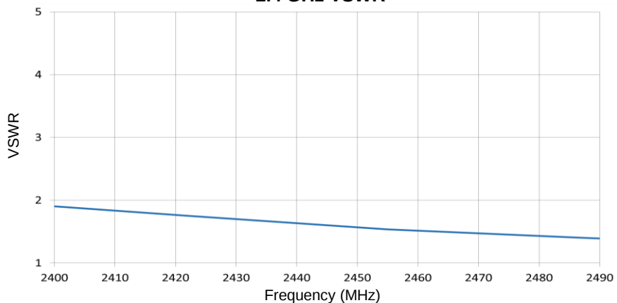
2.4 GHz VSWR
