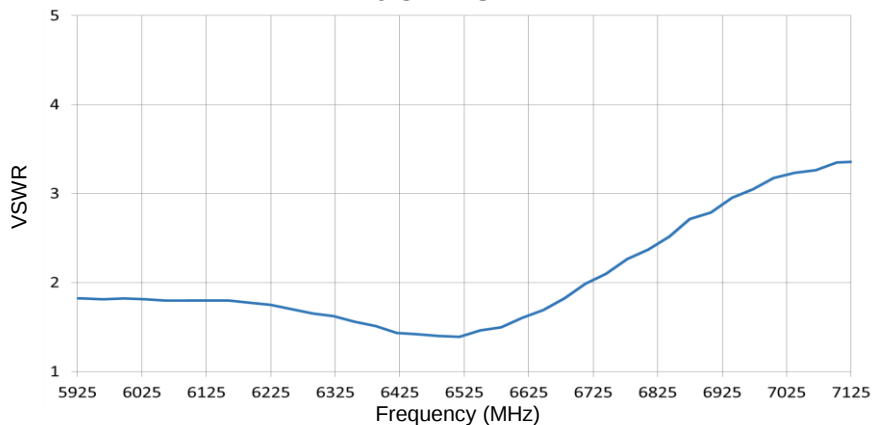
6 GHz VSWR
