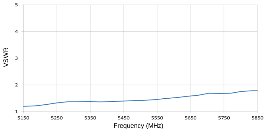
5 GHz VSWR
