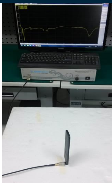
Antenna bent 90°
