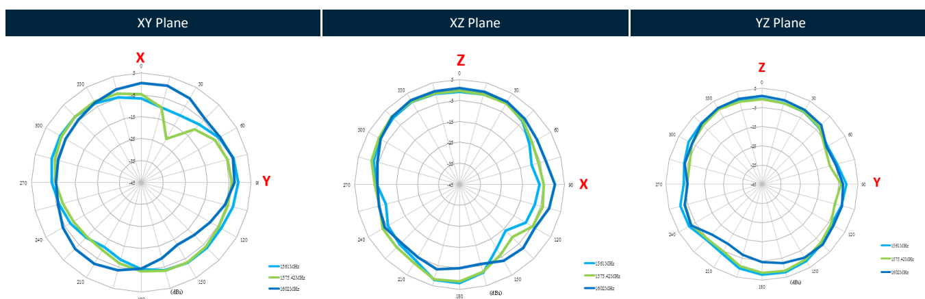
1602MHz
