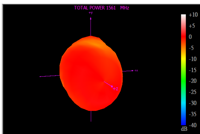
1561MHz
