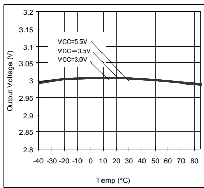
Fig.53 VOUT - Temp
