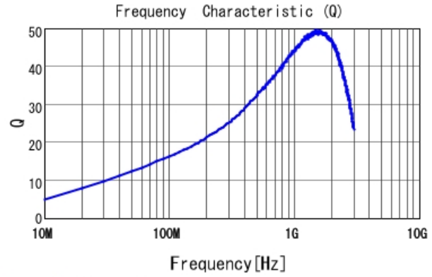
LQG15WH13NG02 Q
