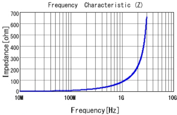
LQG15WH13NG02 |Z|
