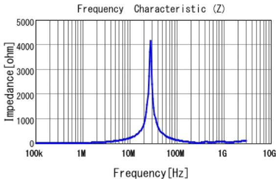
■ FDVE0640-H-3R3M |Z|
