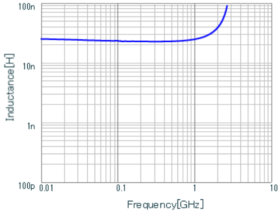
LQG15WH23NG02 L.
