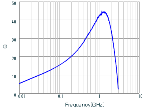
LQG15WH23NG02 Q.
