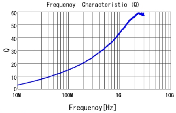
LQW04AN9N8D00 Q
