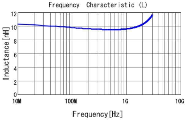
LQW04AN9N8D00 L
