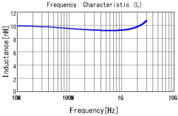
LQW04AN9N4C00 L
