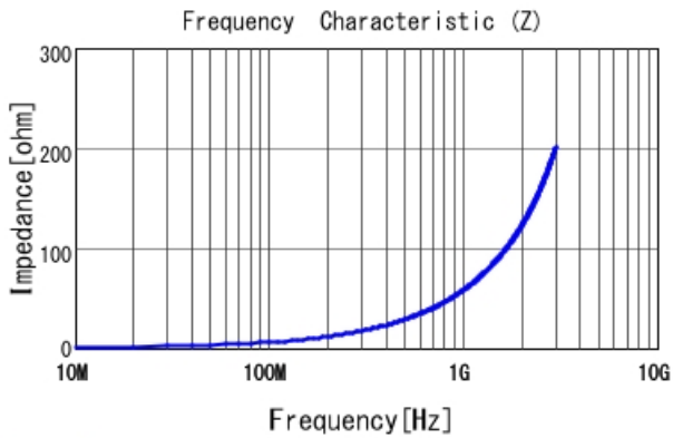
LQW04AN9N4C00 |Z|
