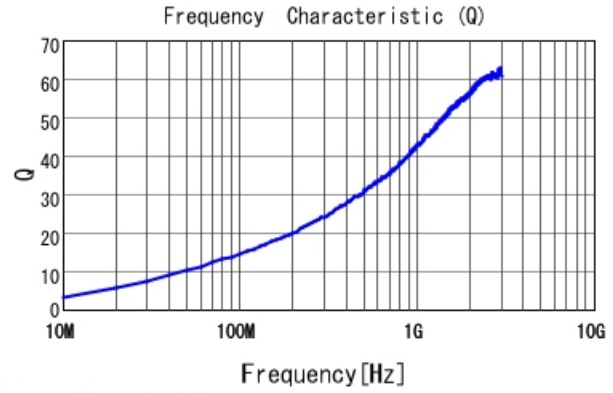
LQW04AN9N4C00 Q
