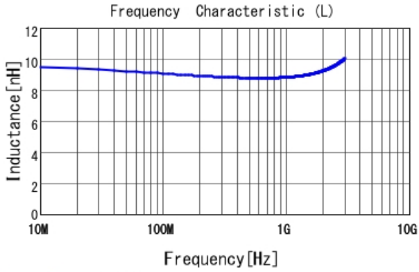
LQW04AN9N0D00 L
