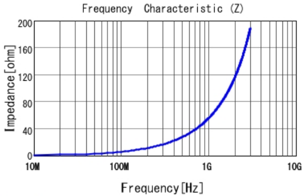
LQW04AN9N0D00 |Z|
