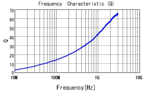
LQW04AN9N0D00 Q
