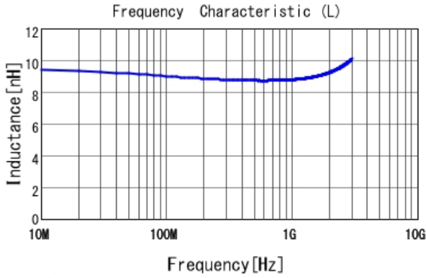
LQW04AN8N9C00 L
