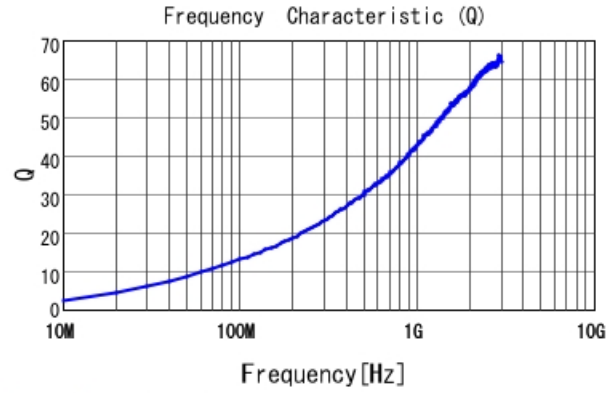
LQW04AN8N9C00 Q
