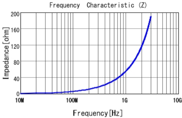
LQW04AN8N9C00 |Z|
