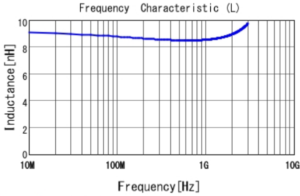
LQW04AN8N7D00 L
