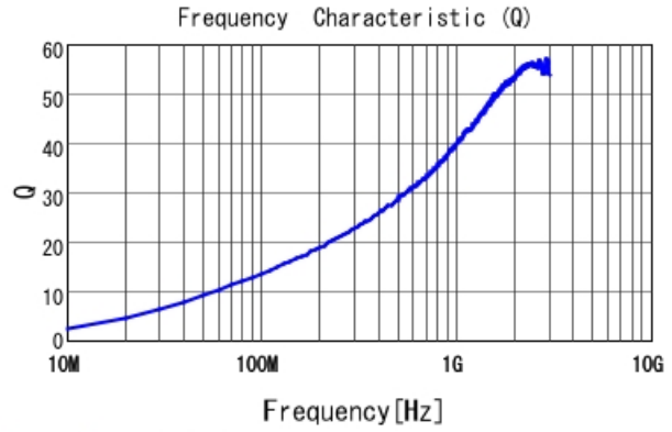
LQW04AN8N7D00 Q
