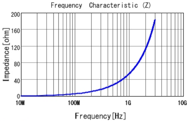
LQW04AN8N7D00 |Z|
