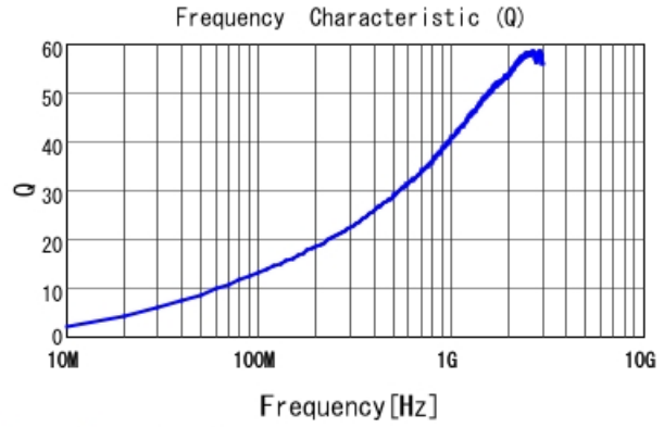
LQW04AN8N5D00 Q
