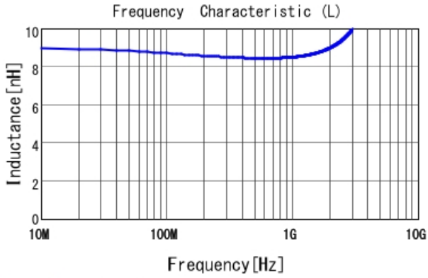
LQW04AN8N5D00 L
