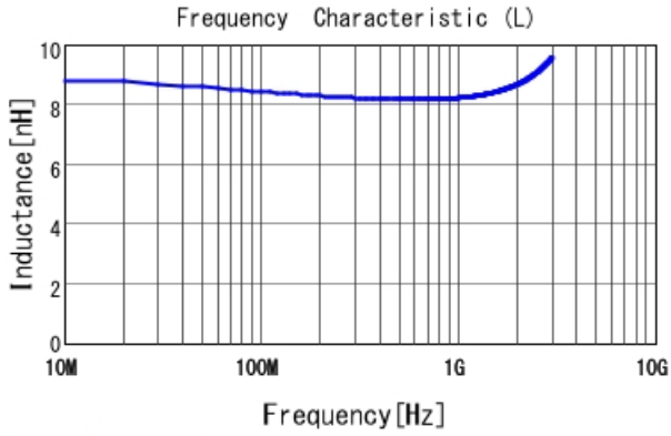
LQW04AN8N3C00 L
