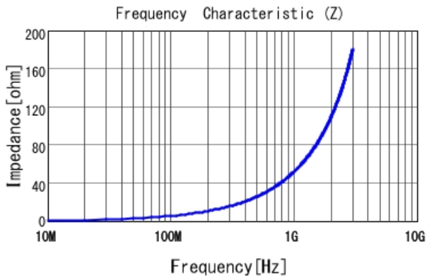
LQW04AN8N3C00 |Z|
