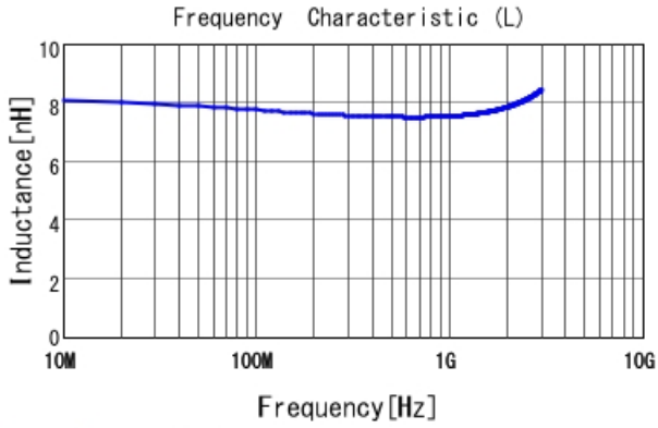
LQW04AN7N7C00 L
