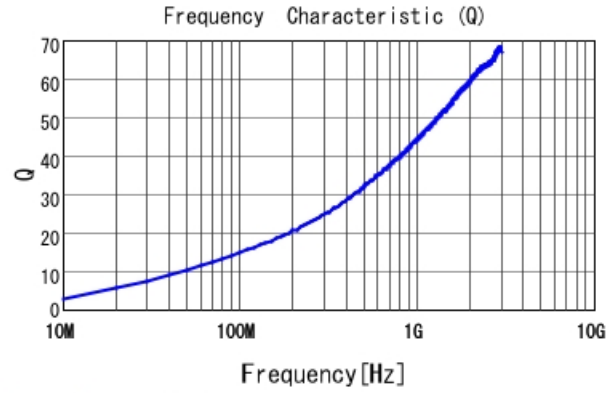
LQW04AN7N7C00 Q
