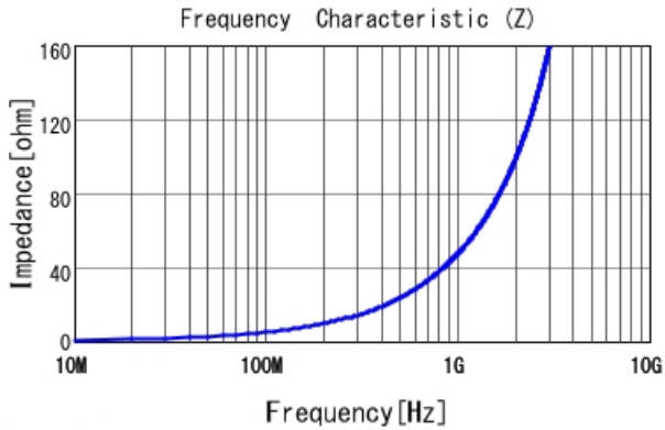
LQW04AN7N7C00 |Z|
