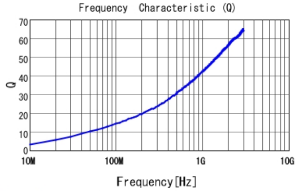
LQW04AN6N6C00 Q
