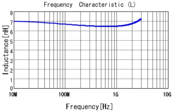
LQW04AN6N6C00 L
