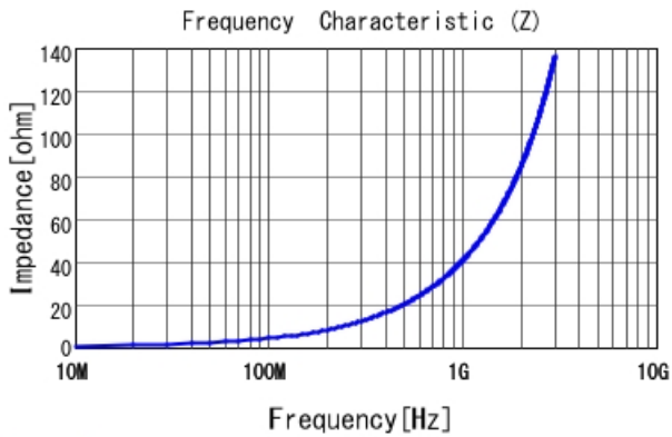
LQW04AN6N6C00 |Z|
