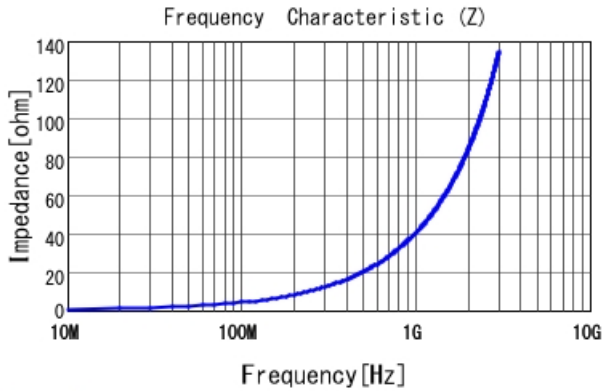
LQW04AN6N5D00 |Z|
