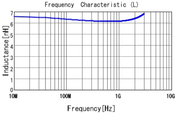
LQW04AN6N3D00 L
