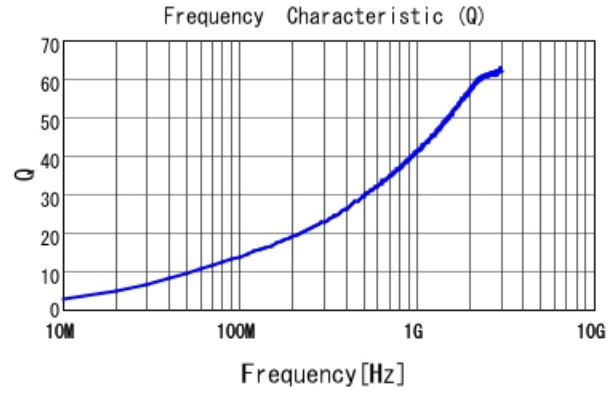
LQW04AN6N0D00 Q
