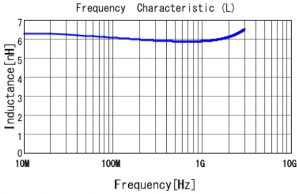
LQW04AN6N0D00 L
