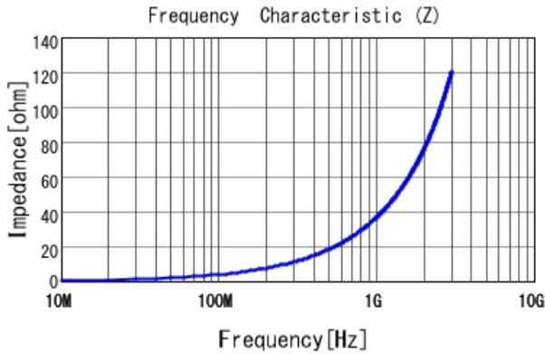
LQW04AN5N9C00 |Z|
