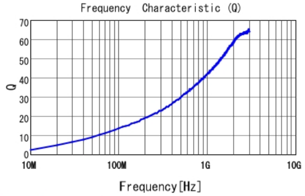
LQW04AN5N9C00 Q
