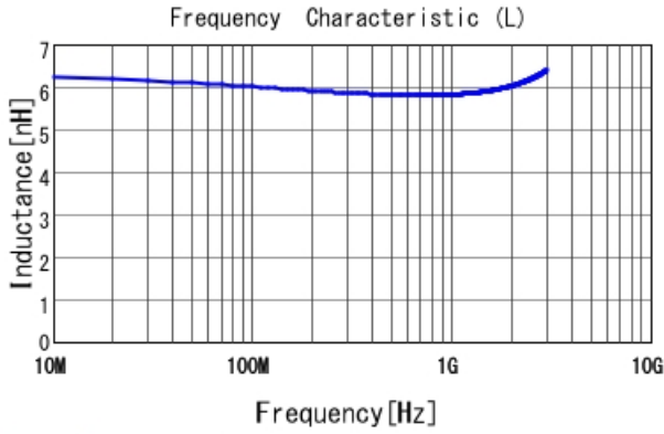
LQW04AN5N9C00 L
