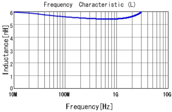
LQW04AN5N5C00 L
