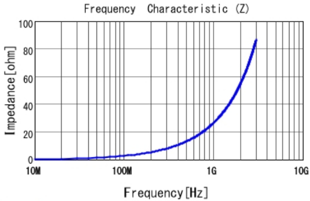
LQW04AN4N2C00 |Z|
