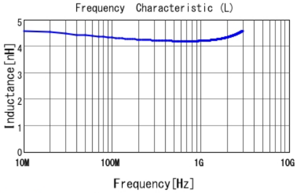
LQW04AN4N2C00 L
