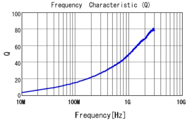
LQW04AN4N2C00 Q
