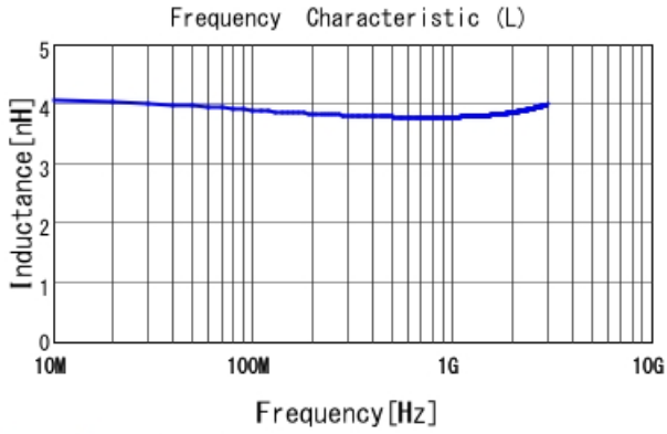
LQW04AN3N9C00 L
