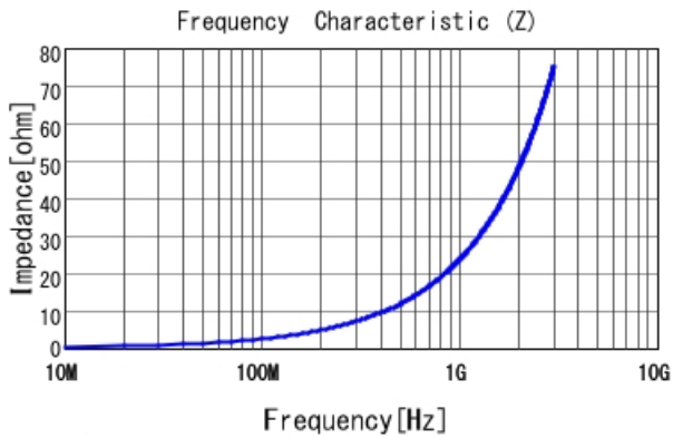
LQW04AN3N9C00 |Z|
