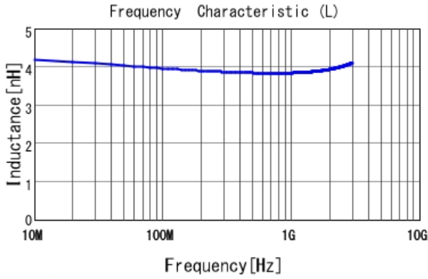
LQW04AN3N8D00 L
