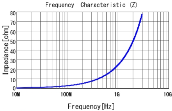
LQW04AN3N8D00 |Z|
