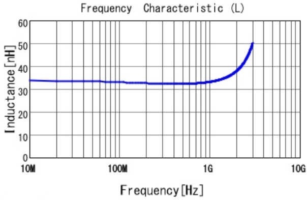
LQW04AN33NH00 L
