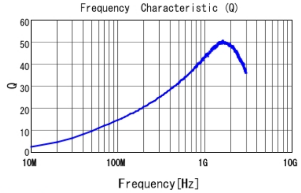
LQW04AN33NH00 Q
