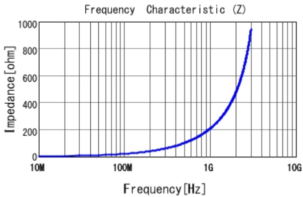
LQW04AN33NH00 |Z|
